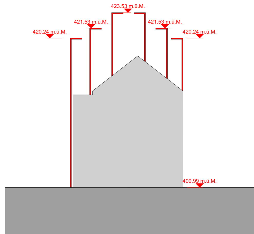
Schnitt
