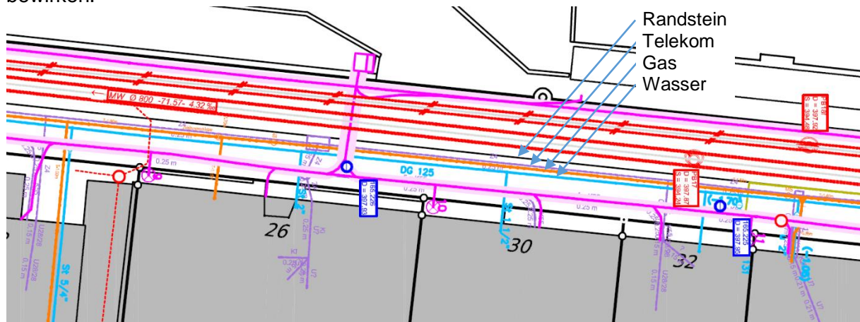
Abb: Leitungskataster
